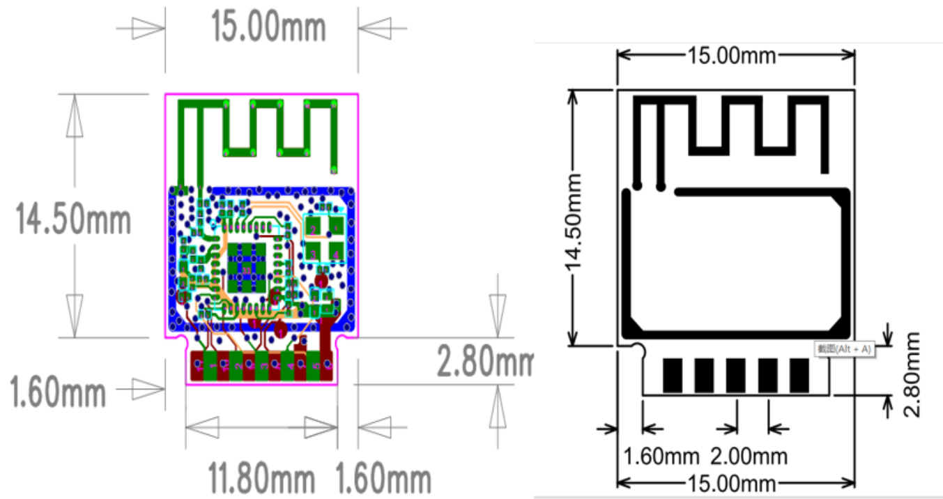
图 4 模组尺寸
