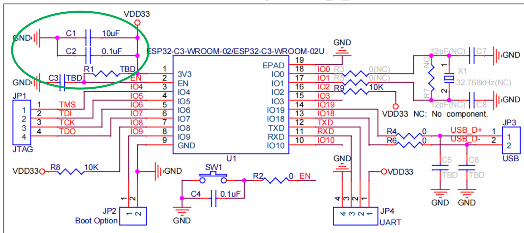
图 7 应用电路图
