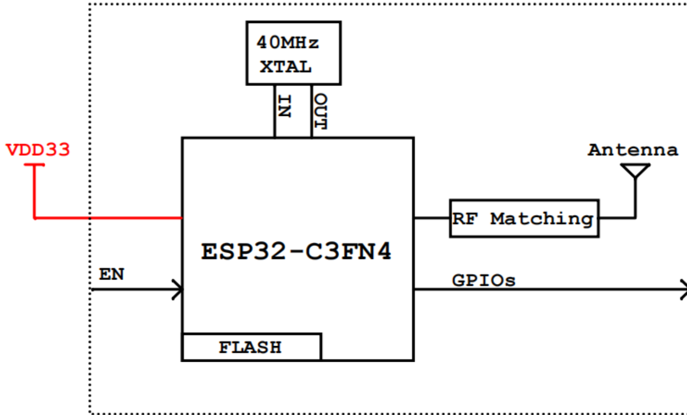
图 1 硬件框图
