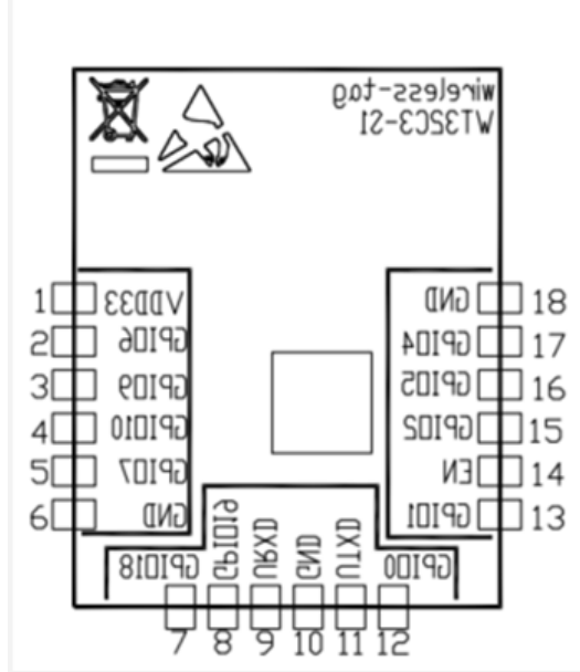
图 3 交互物体引脚图
