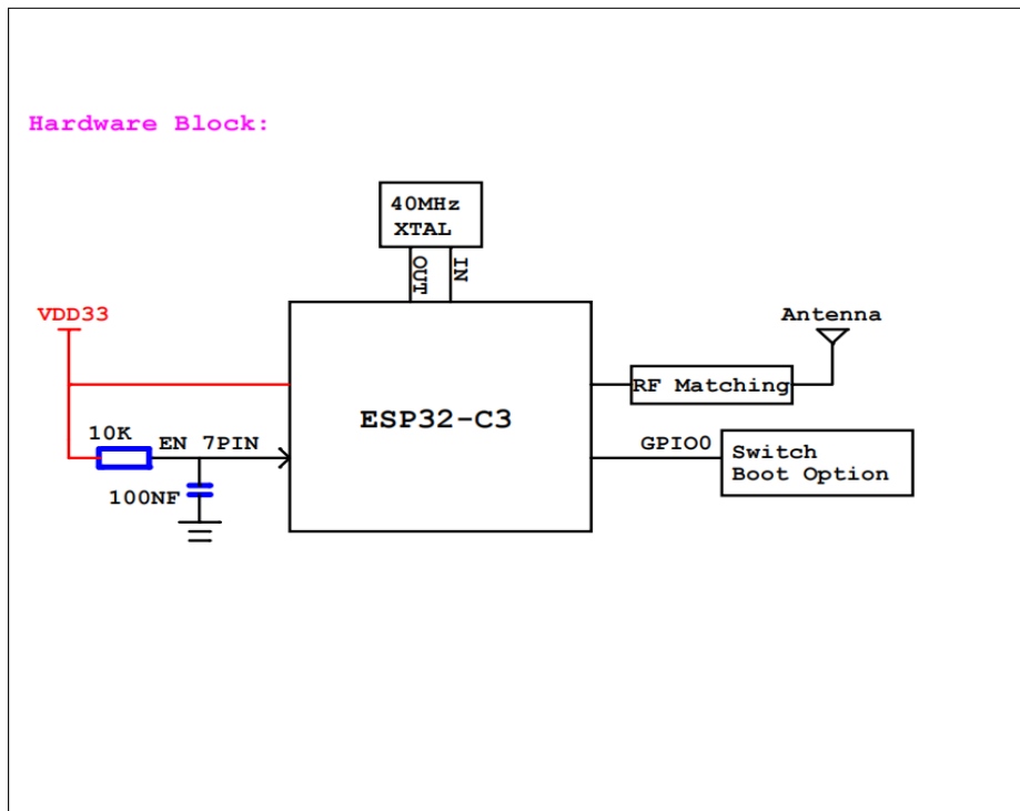
图 1 硬件框图
