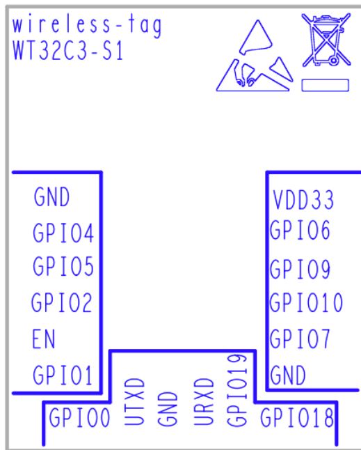
图 2 产品实物引脚图
