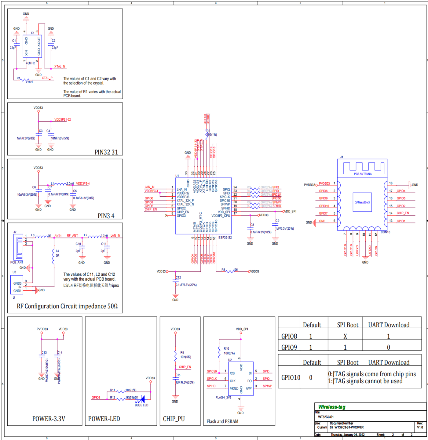
图 6 模组原理图
