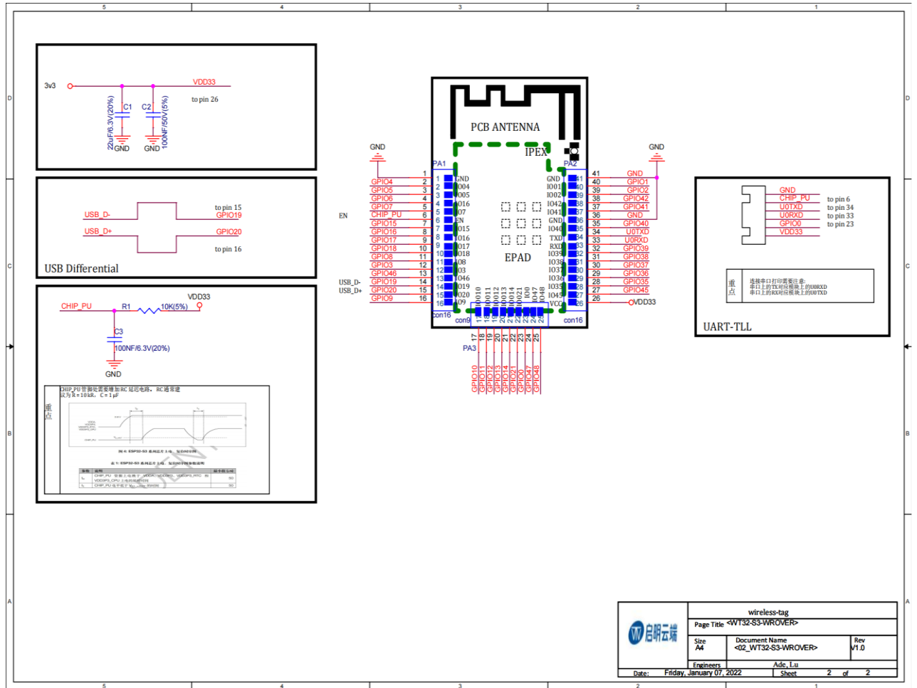
图 5 应用电路图
