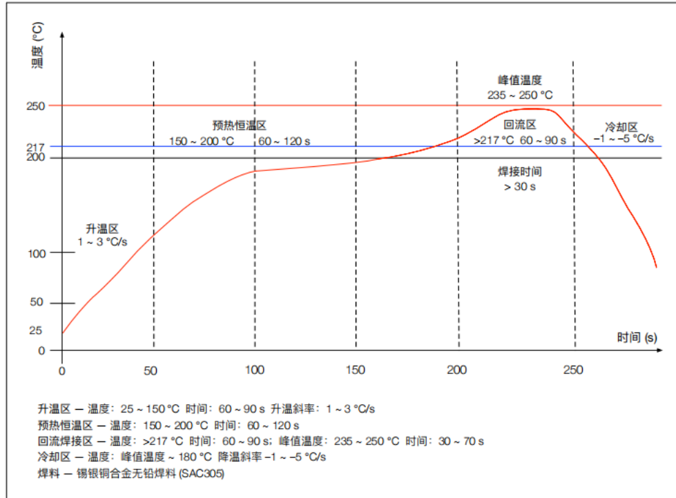
图 4 回流焊曲线
