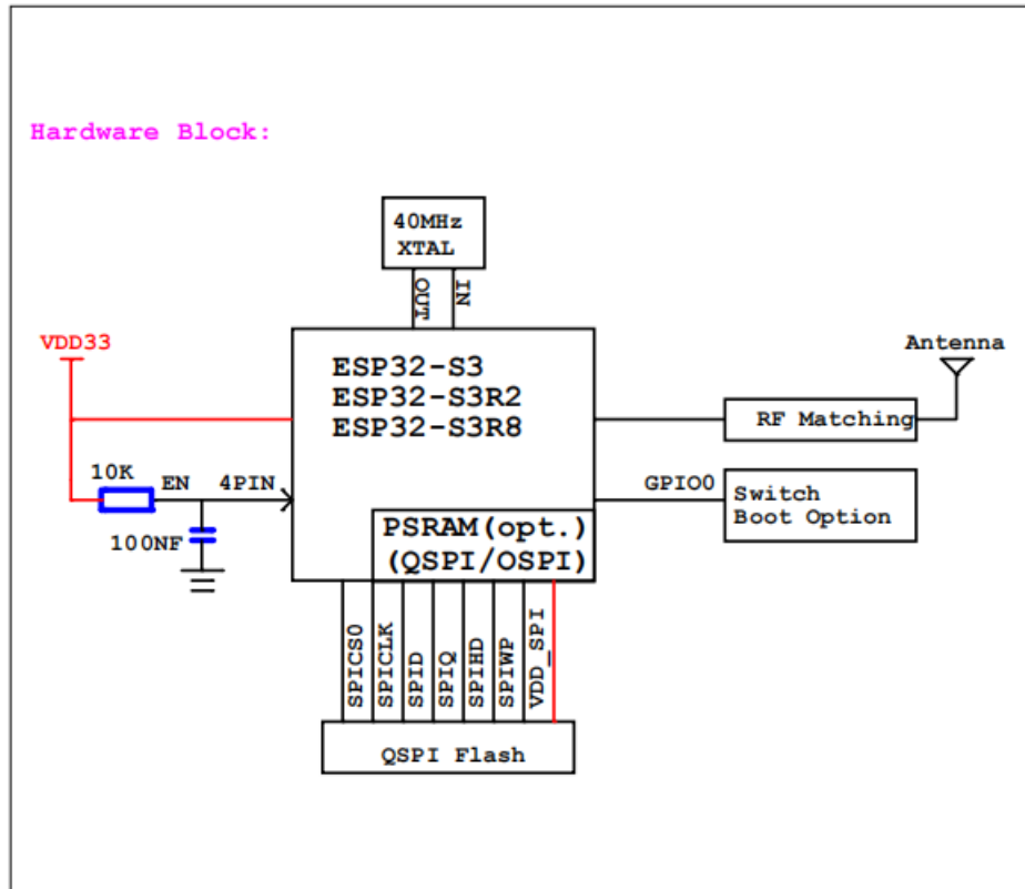
图 1 硬件框图
