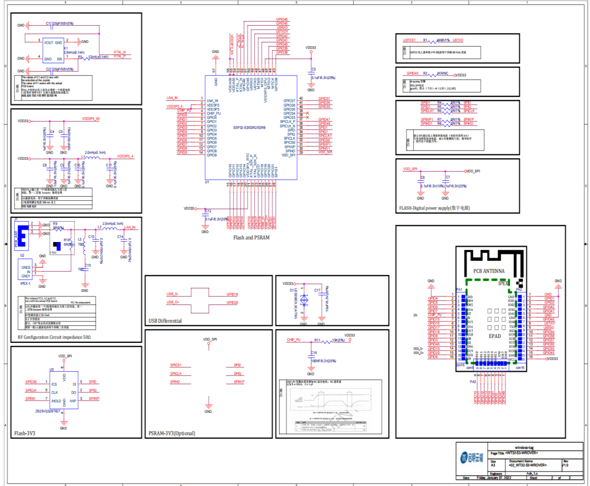
图 5 模组原理图
