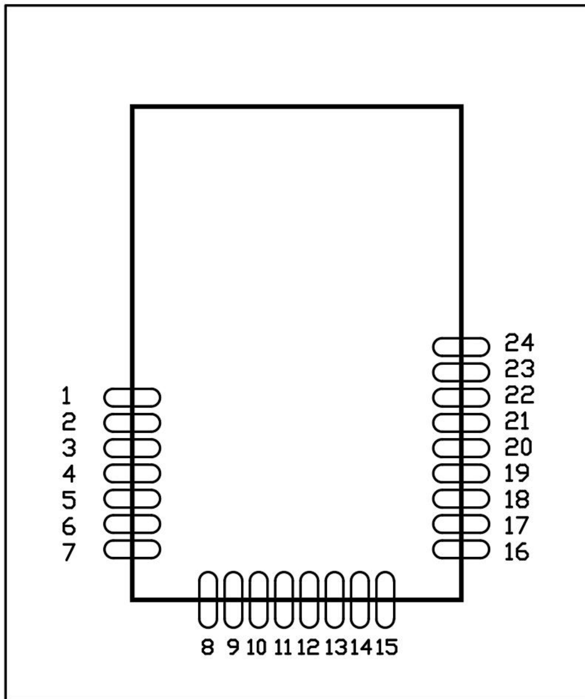
图 4 引脚俯视图
