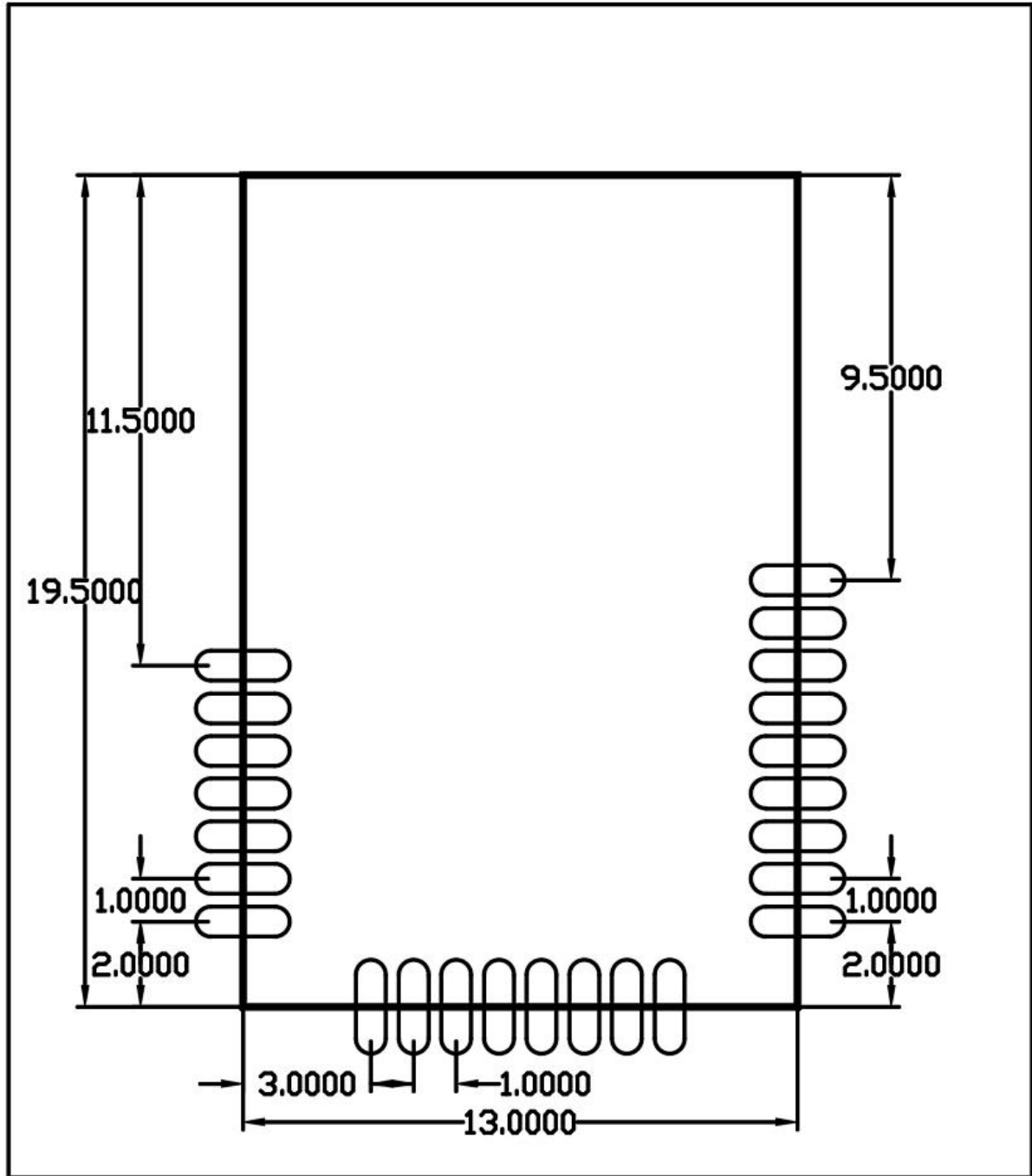
图 1 模组尺寸图
