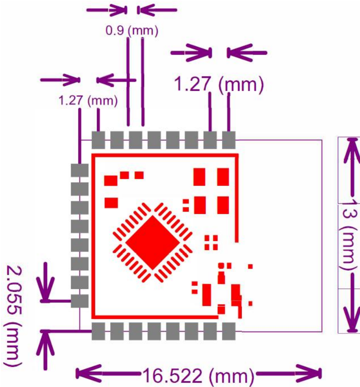
图 1 模组尺寸图
