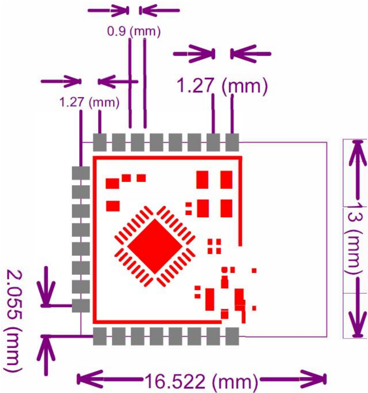
图 1 模组尺寸图
