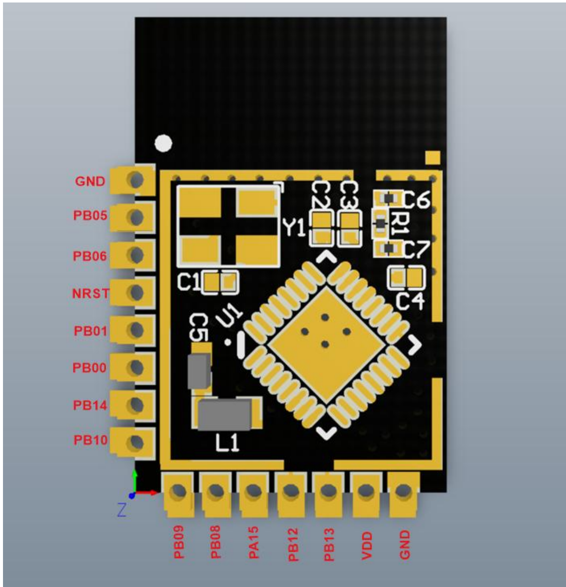
图 2 引脚正视图
