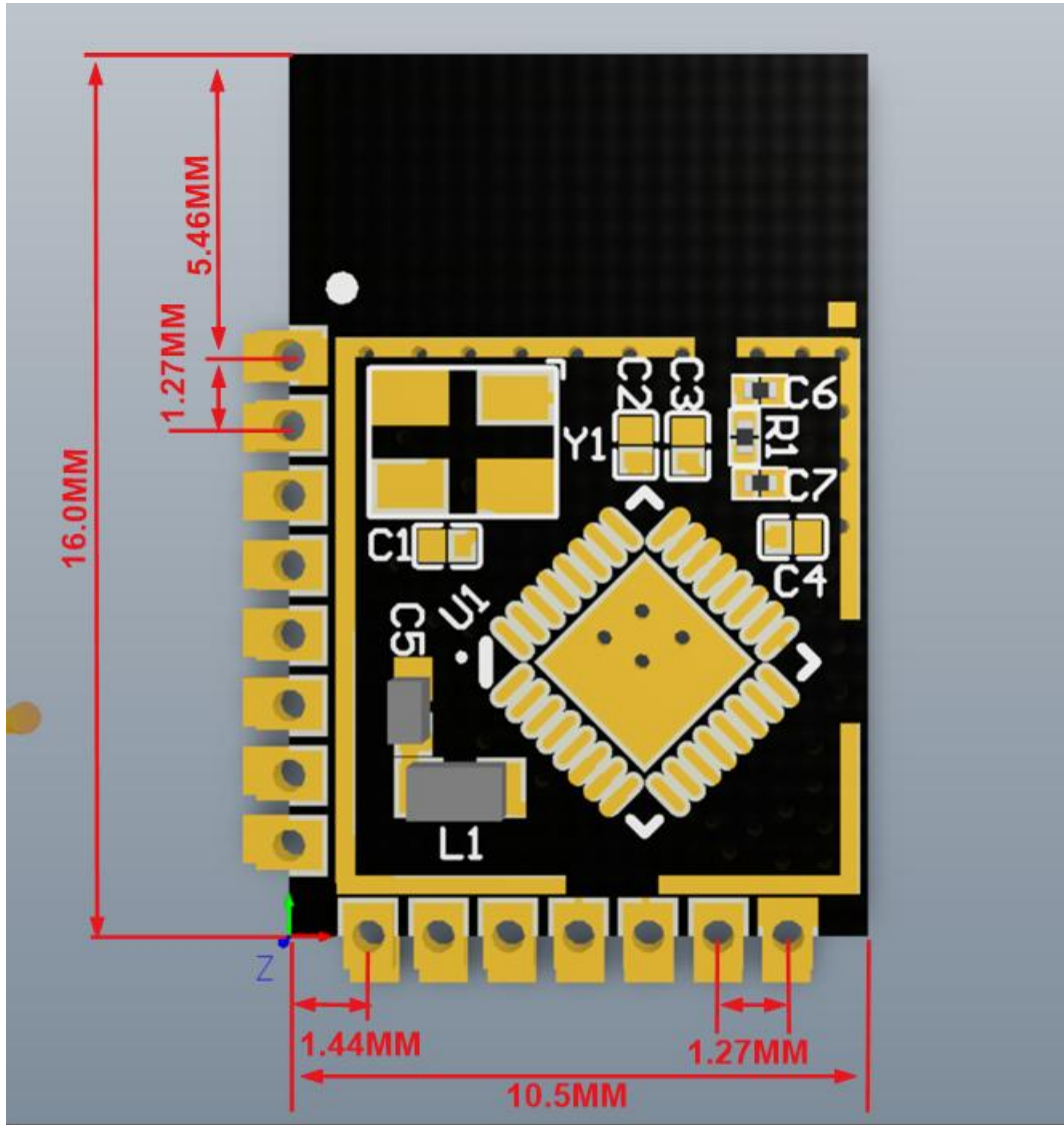
图 1 尺寸图
