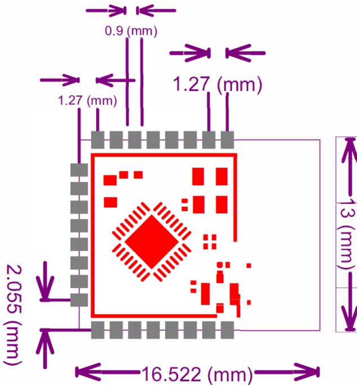
图 1 模组尺寸图
