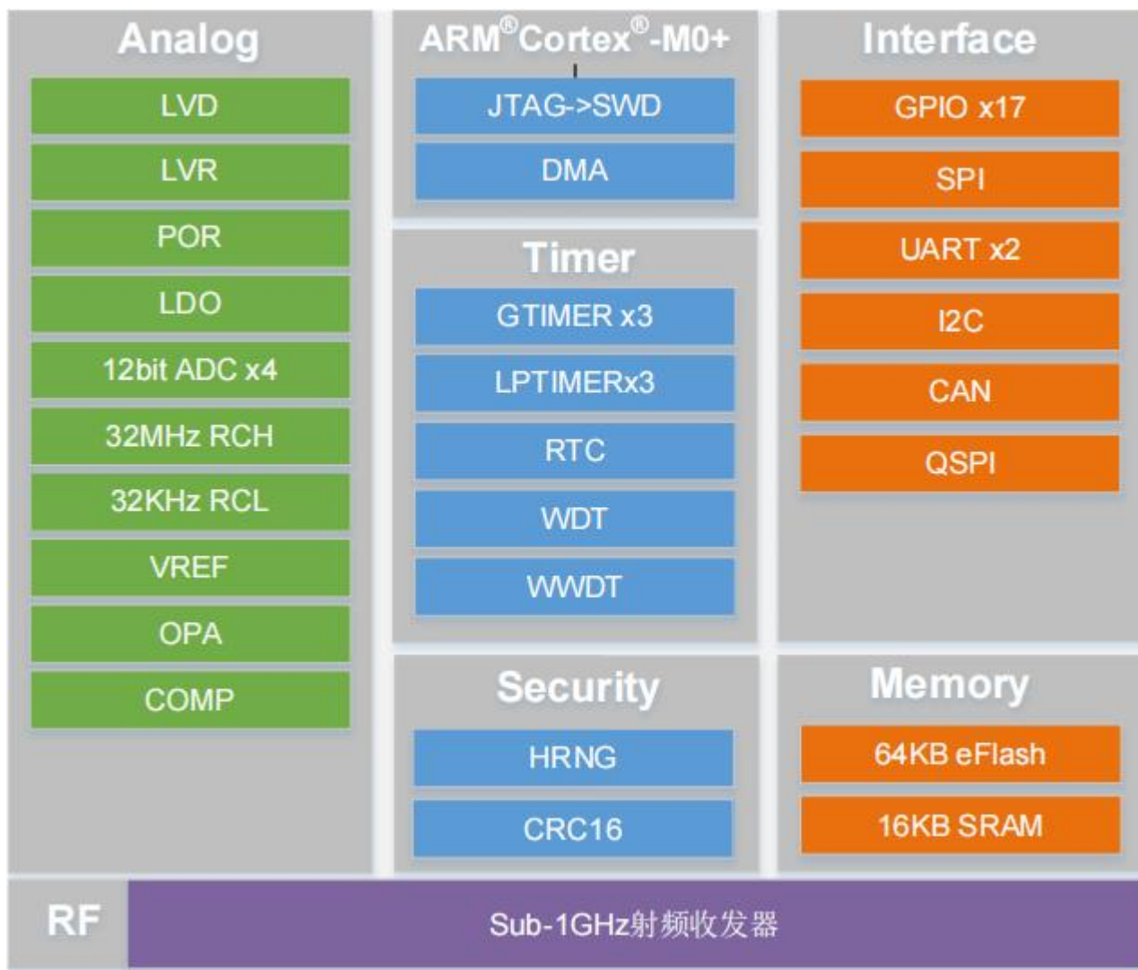
图-1 系统框图
