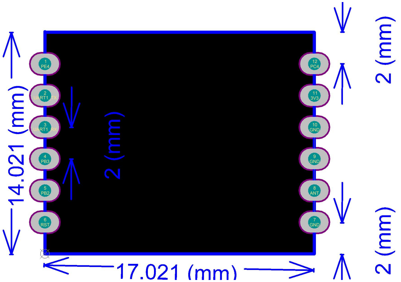
图-2 产品尺寸图 (管脚之间间距2.0mm)
